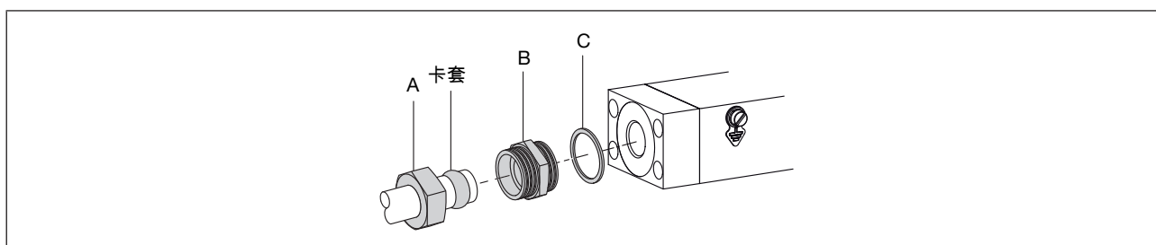
图 7: 管道上的螺母和卡套
