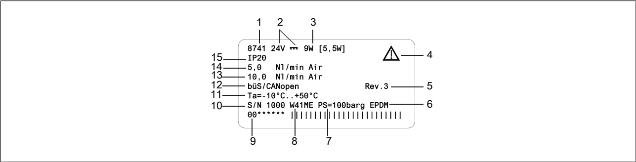
图 1: 8741 型铭牌示例
