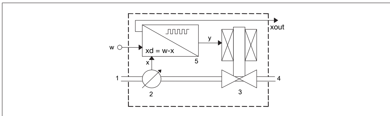
图 18: 带调节阀的 MFC 功能图
