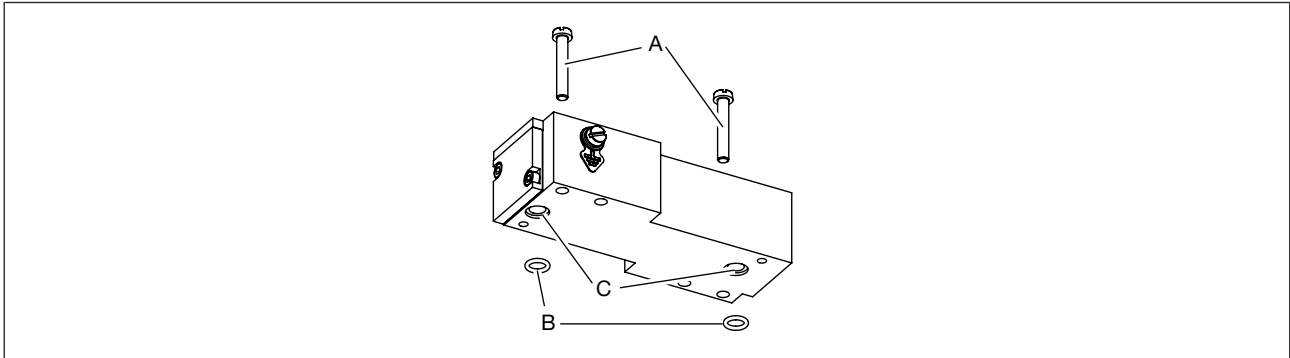
图 14: 使用螺栓和 O 型圈密封件的法兰连接
