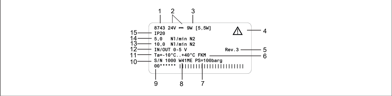
图 1: 8743 型铭牌示例
