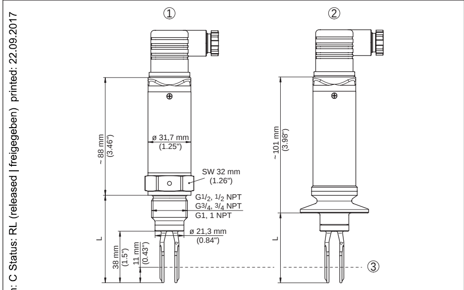
Abb. 34: LEVEL SWITCH 8110, Hochtemperaturausführung
