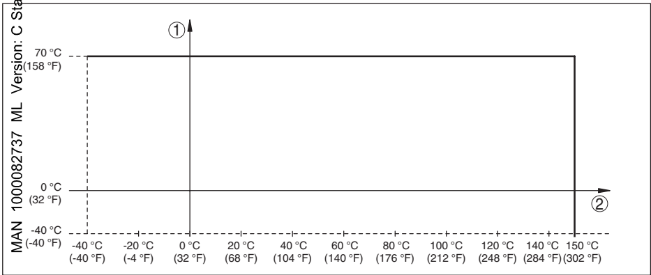
Abb. 31: Abhängigkeit Umgebungstemperatur zu Prozesstemperatur
