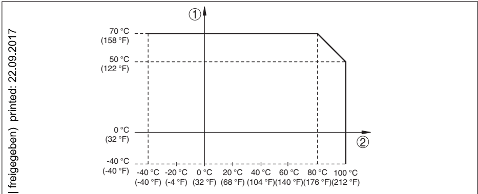
Abb. 30: Abhängigkeit Umgebungstemperatur zu Prozesstemperatur
