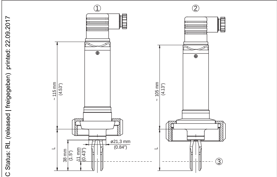
Fig. 35: LEVEL SWITCH 8110, version haute température
