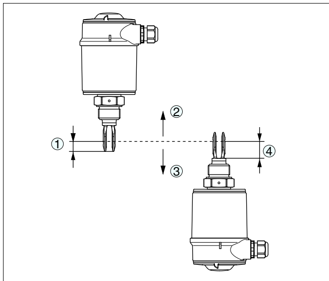
Abb. 2: Einbau senkrecht
