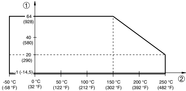
Fig. 25: Température process - pression process avec position du commutateur 0,5 g/cm³ (commutateur inversion de la sensibilité)
