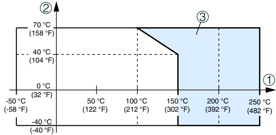
Fig. 23: Température ambiante - température process
