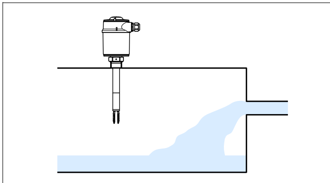
Abb. 8: Einströmendes Füllgut
