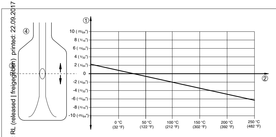
Abb. 22: Einfluss der Prozesstemperatur auf den Schaltpunkt
