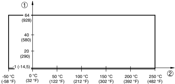
Fig. 24: Température process - pression process avec position du commutateur 0,7 g/cm³ (commutateur d'inversion de la sensibilité)
