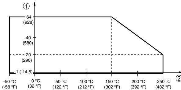
Abb. 27: Prozesstemperatur - Prozessdruck bei Schalterstellung 0,5 g/cm 3 (Empfindlichkeitsumschalter)
