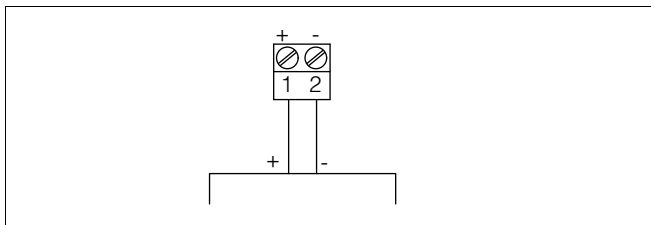
Abb. 11: Anschlussplan Einkammergehäuse
