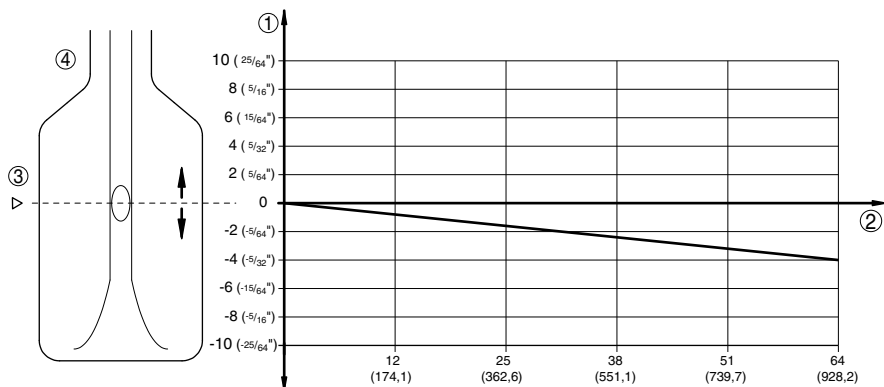
Décalage du point de commutation en mm (in) Pression process en bar (psig) Point de commutation avec conditions de référence (rainure) Lames vibrantes
