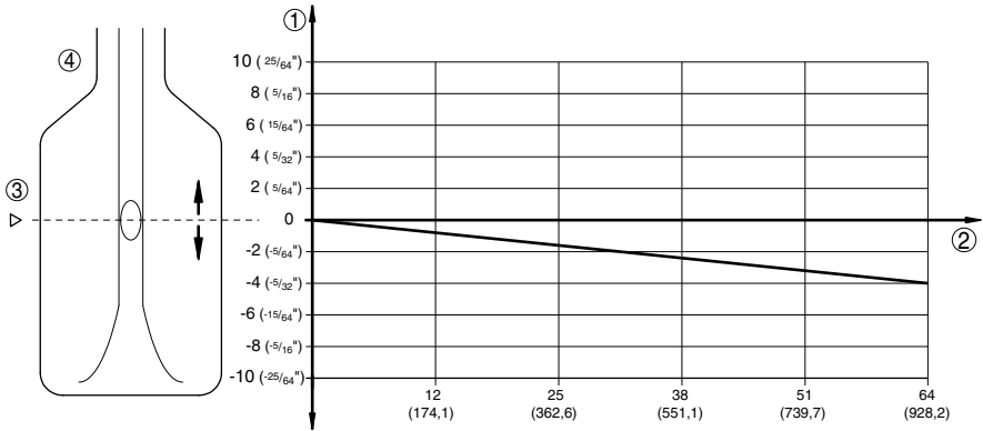
Abb. 24: Einfluss des Prozessdrucks auf den Schaltpunkt
